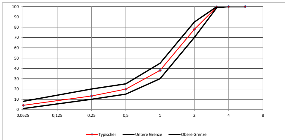
Richtungsweisende Siebkurve (w/w%)
